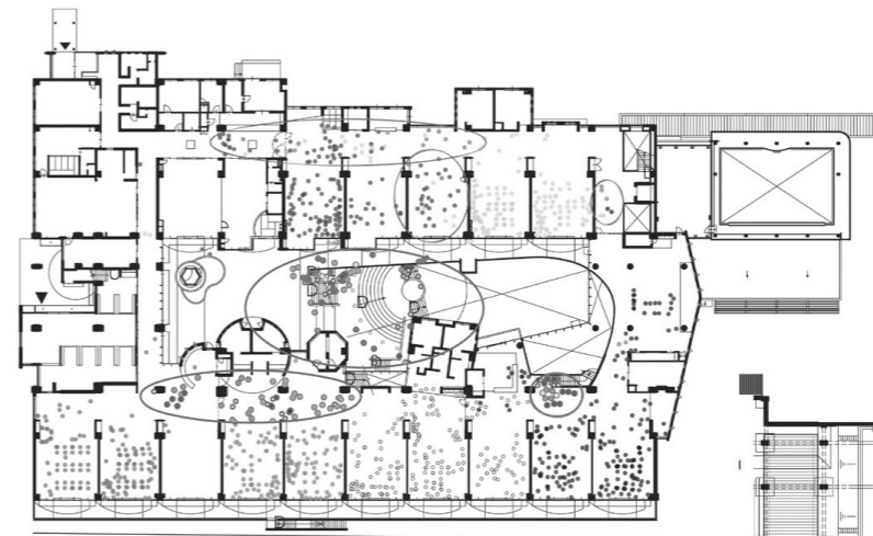
2F平面図
